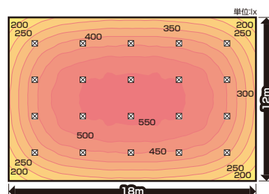
水平面照度分布図 計算面高さ0m
