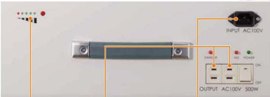
残量計 AC100V出力コンセント(2口) 電源 2口あわせて、消費電力500Whまで使用できます。 電源を入れるとランプが点灯します。
